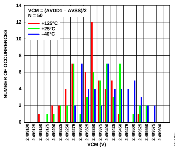
Figure 45. VCM Output Voltage Distribution, V_{CM} = (AVDD1 - AVSS)/2
