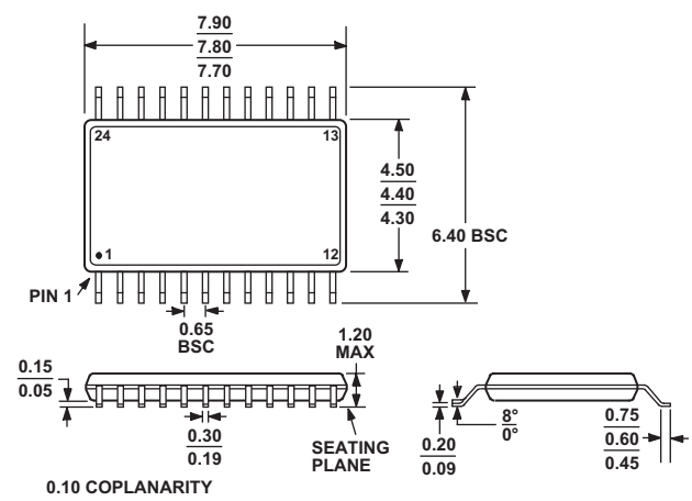
图 33. 24 引脚超薄紧缩小型封装 [TSSOP] (RU-24)
