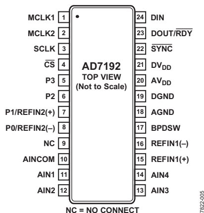
图 5. 引脚配置
