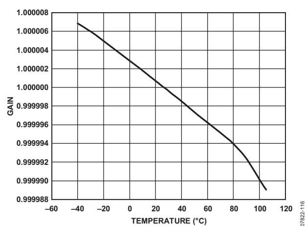
图 16. 增益误差 (增益 = 1)
