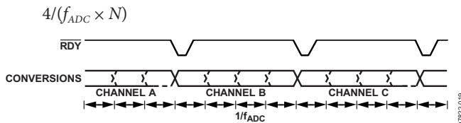
图 28. 通道序列器
