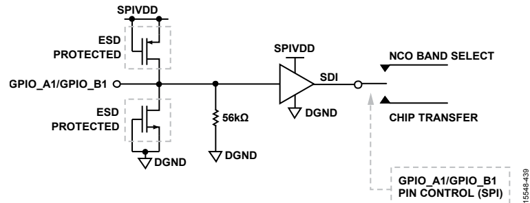
Figure 41. GPIO_A1/GPIO_B1
