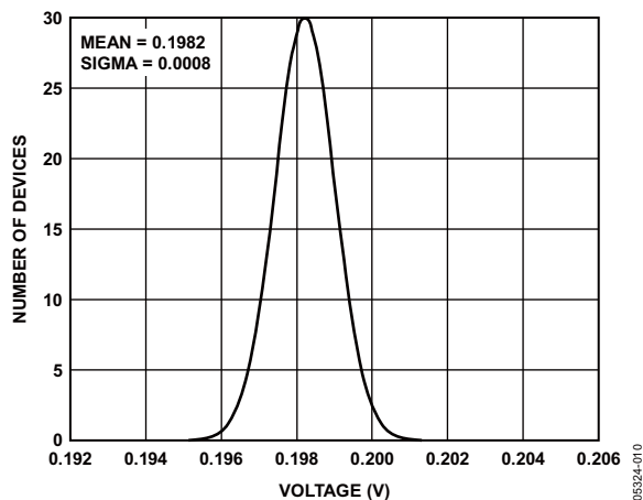
图10. 范围4输出激励电压分布, V_{DD} = 3.3\text{ V}
