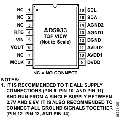
图3. 引脚配置
