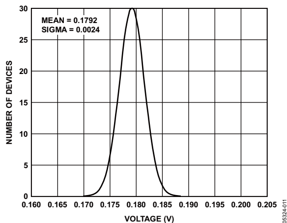
图11. 范围4直流偏置分布, V_{DD} = 3.3\text{ V}
