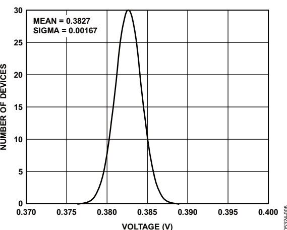
图8. 范围3输出激励电压分布, V_{DD} = 3.3\text{ V}
