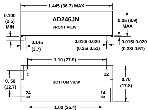
AD246JN Package
