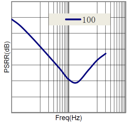
PSRR
