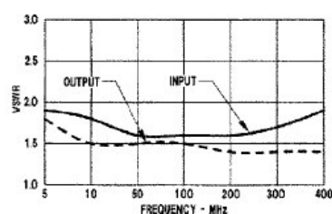
VSWR
