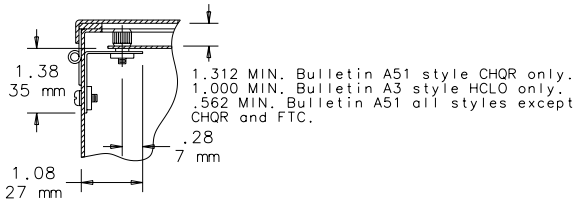
DETAIL Y
