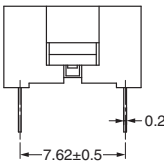
Flat Actuator
