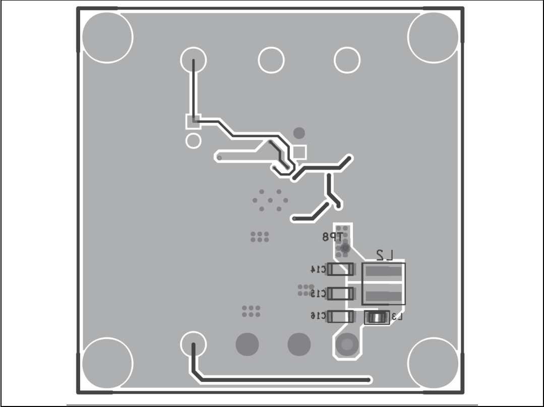
Figure 56. Bottom layer
