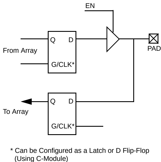
Figure 5 • I/O Module
