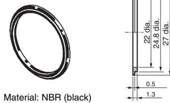
25-dia. Ring A22Z-R25
