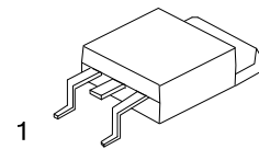
TO-263
