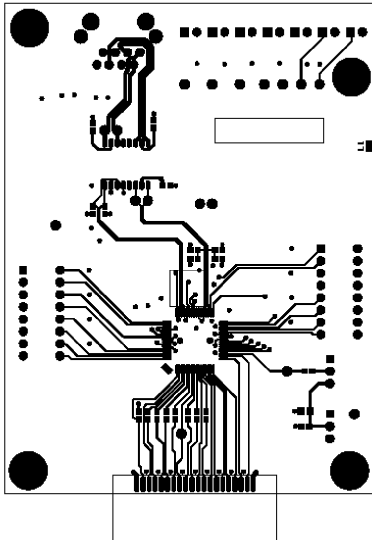
Top Layer
