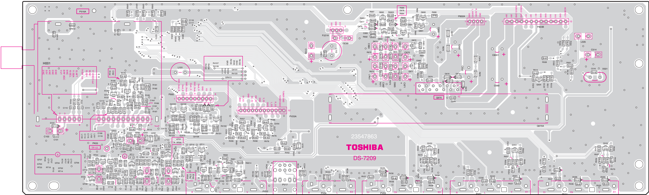
TN AV BOARD PD2224A1 (U003A) BOTTOM (FOIL) SIDE
