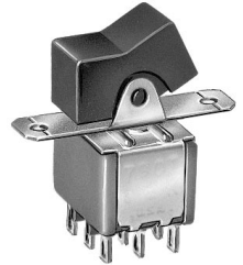
7301J1ZQE2 3PDT
