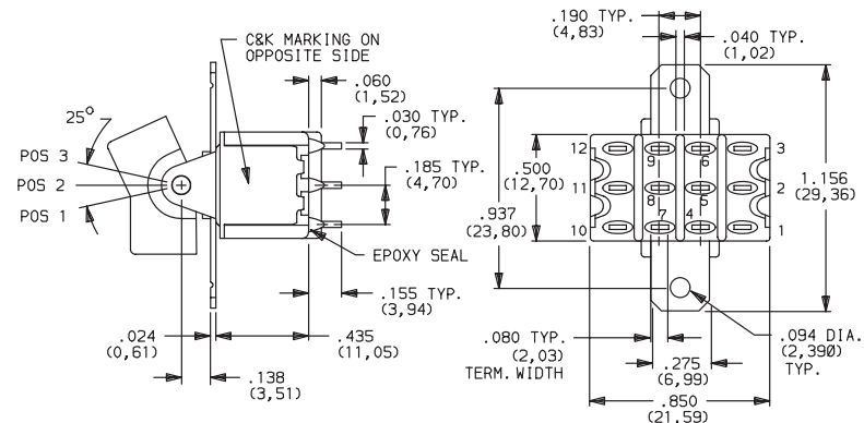
7401J1ZQE2 4PDT
