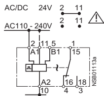
Flashing, starting with interval (D)
