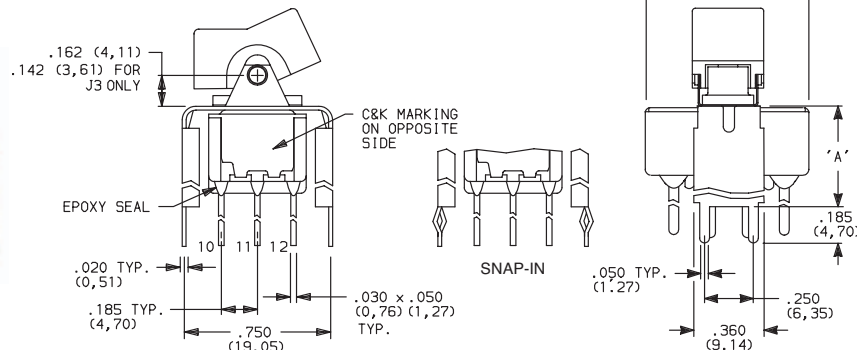
7401J1_BE2 4PDT
