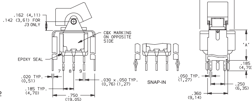
7301J1_BE2 3PDT
