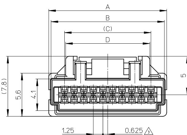
ターミナル装着図 TERMINAL ASSEMBLY DRAWING
