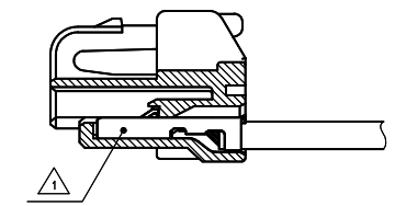
ターミナル装着図 TERMINAL ASSEMBLY DRAWING
