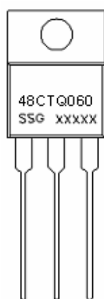
48CTQ060
