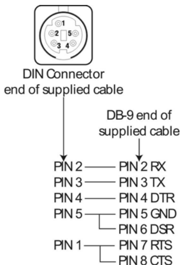
DIN to DB-9 Cable
