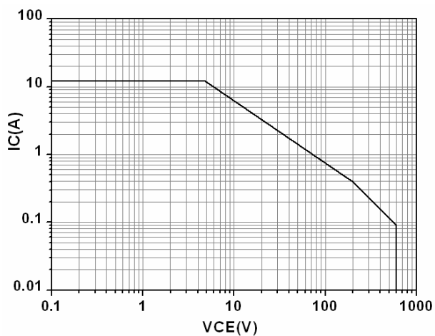
SOA
