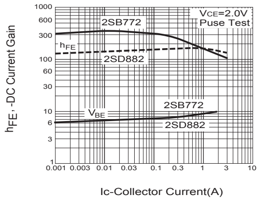
F7. h_{FE} , V_{BE} - I_C
