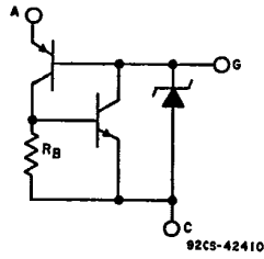
Fig. 23—Equivalent circuit.
