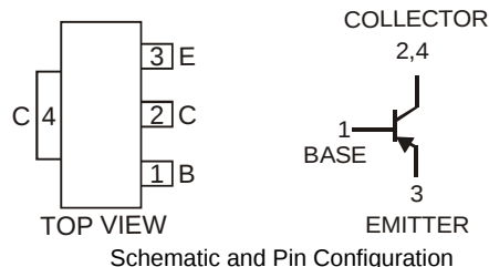
SOT89-3L
