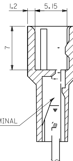
ターミナル装着状態図 TERMINAL ASSEMBLY DRAWING
