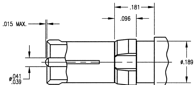
Receptacle Interface
