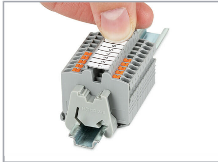
Einrasten eines Beschriftungsstreifens (2009-110) in die Beschriftungsaufnahme
