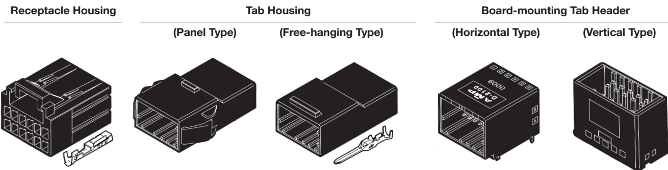
Receptacle Contact
