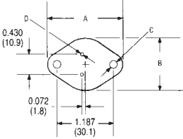
TO-3
