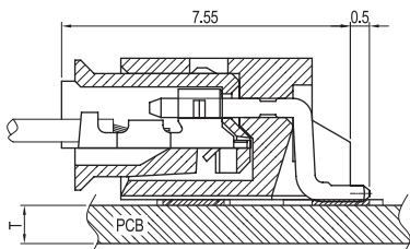
PCB ASS'Y
