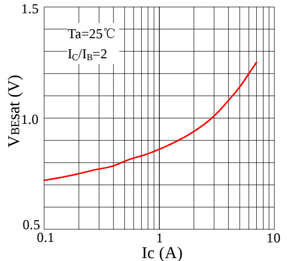
Fig6 VBESat-IC
