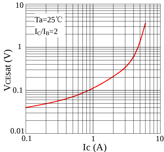
Fig5 VCESat-IC
