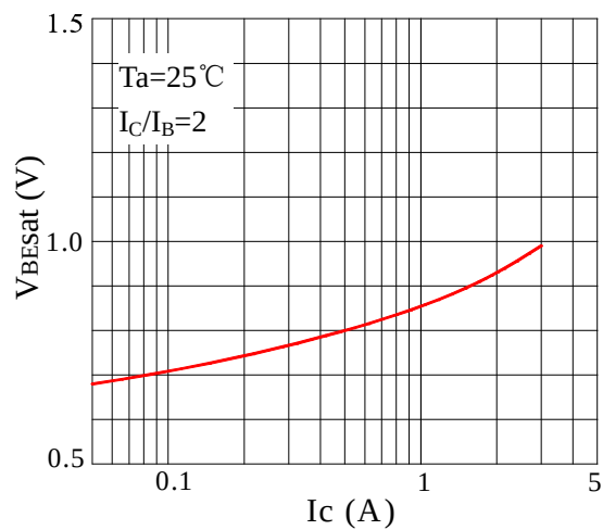
Fig6 VBESat-IC
