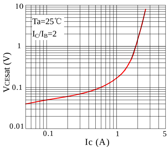
Fig5 VCESat-IC
