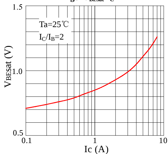
Fig6 VBEsat-IC
