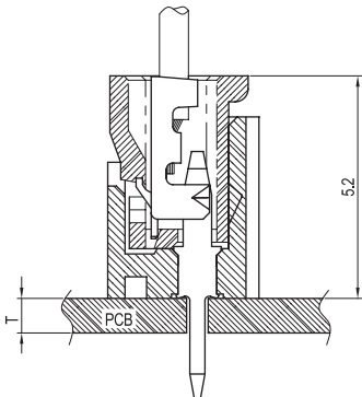
PCB ASS'Y
