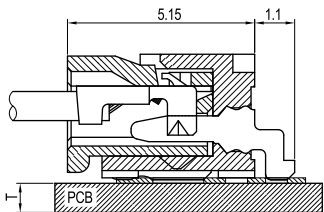
PCB ASS'Y결합도
