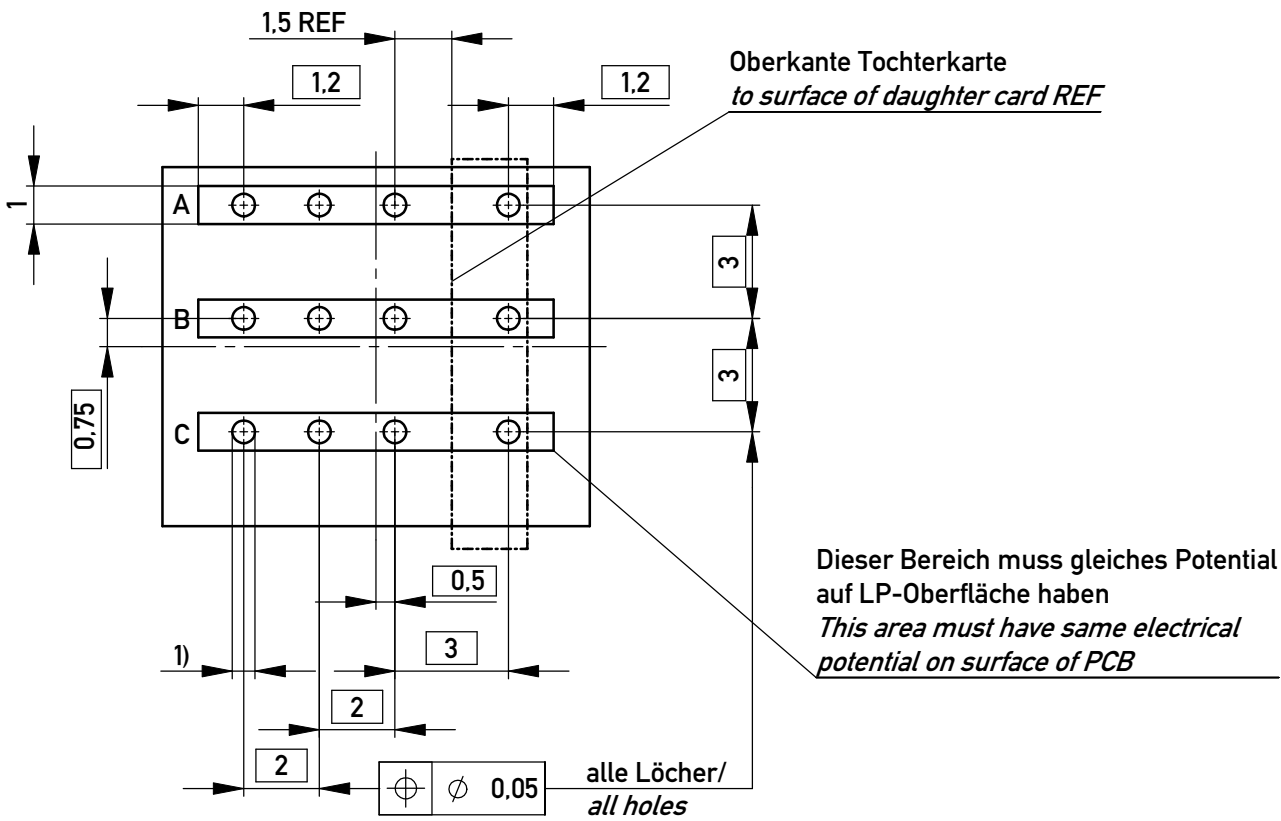
Lochbild für Leiterplatte / Board hole pattern
