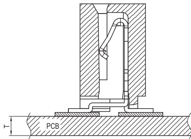
PCB ASS'Y
