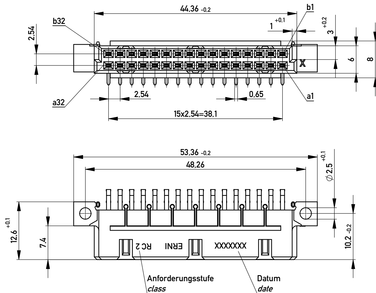
Bestückungsplan / contact layout
