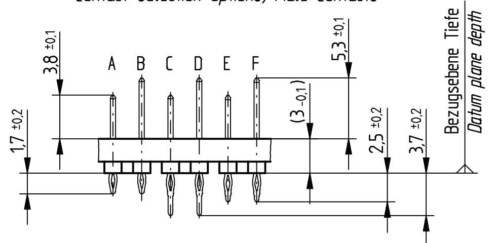
Kontaktversionen, Messerkontakte Contact Selection Options, Male Contacts
