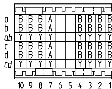
Bestückungsplan - contact layout
