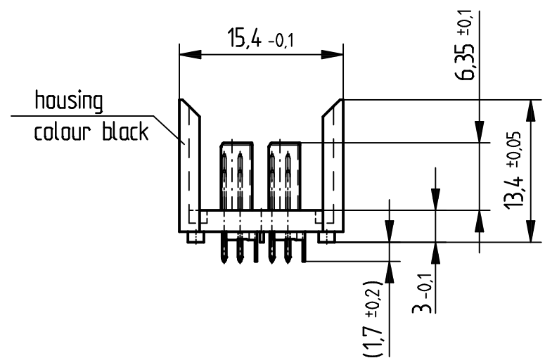
Kontaktversionen, Messerkontakte Contact Selection Options, Male Contacts
