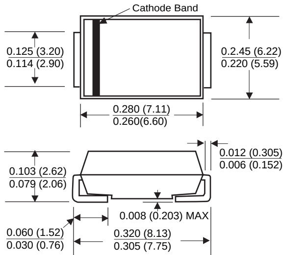
DO-214AB (SMC J-Bend)
