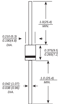
DO-201AD
