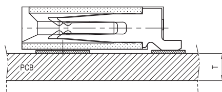
PCB ASS'Y
