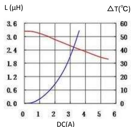
9. 0415CDMCCDS-3R3MC
