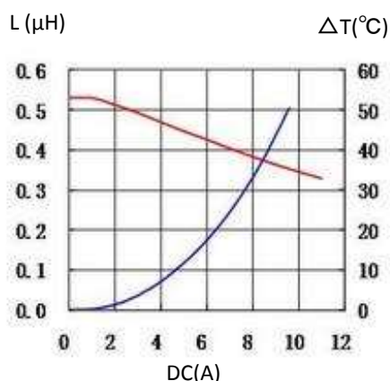
4. 0415CDMCCDS-R56MC
