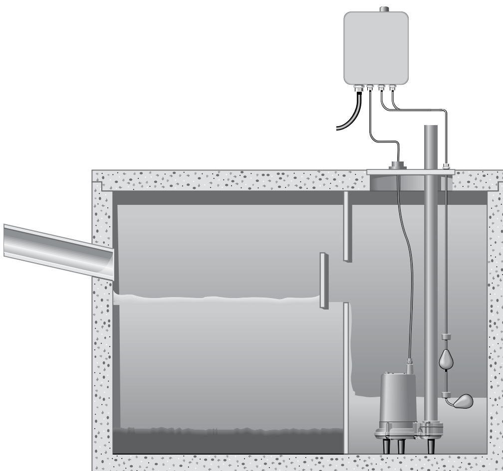
Installation typique à une pompe triphase
