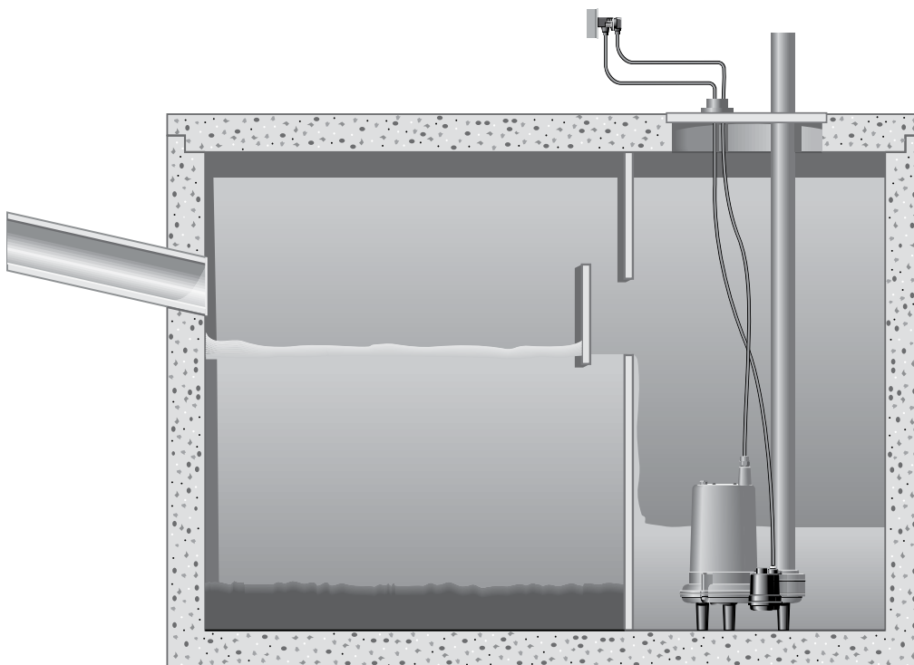
Installation typique à une pompe seule phase
